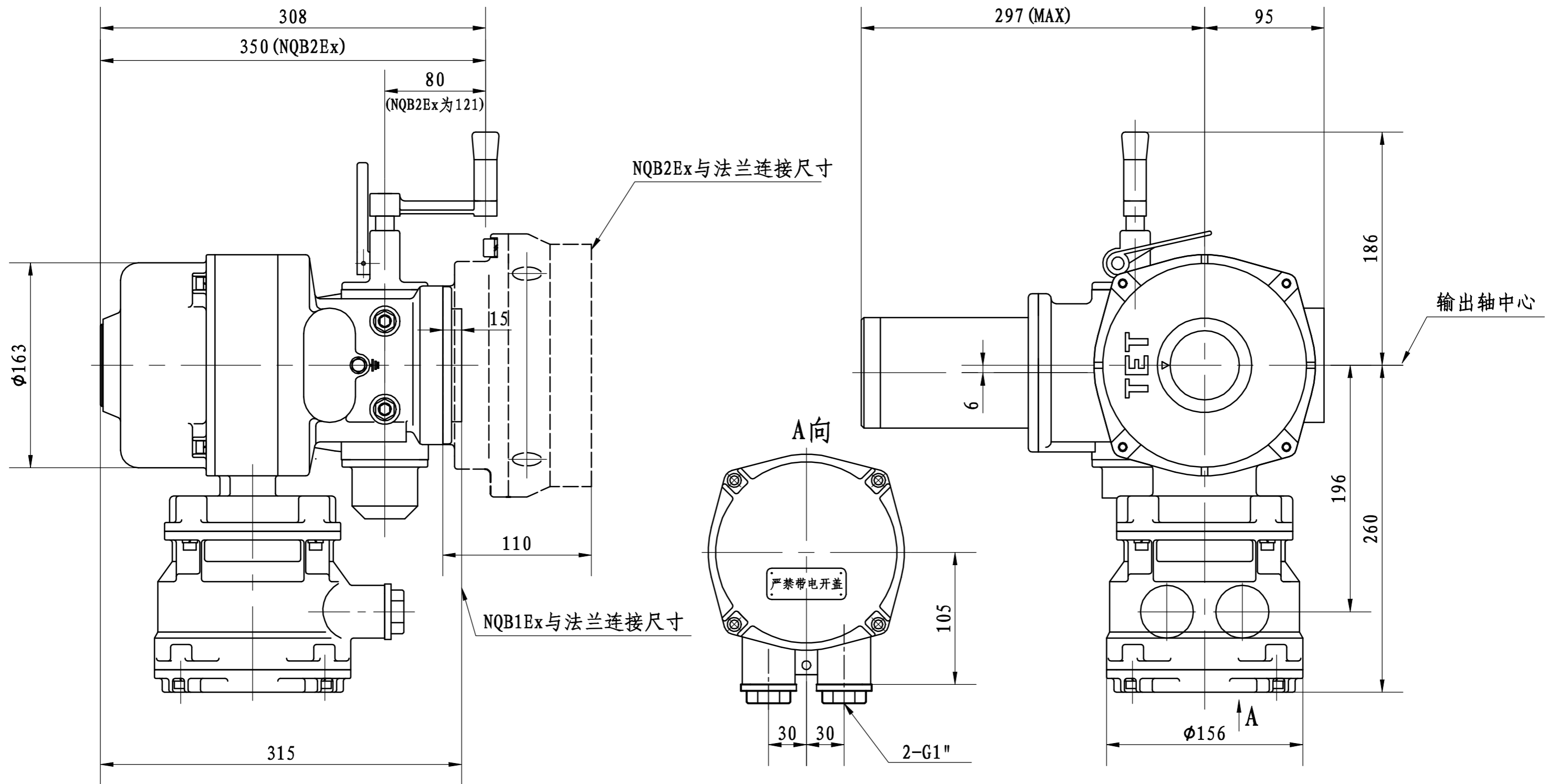
NQB1Ex、NQB2Ex防爆型产品外形尺寸图
